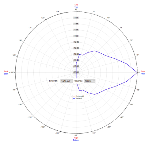
Polardiagramm 4000Hz
