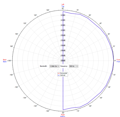
Polardiagramm 500Hz
