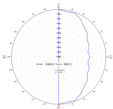
Polardiagramm 500Hz
