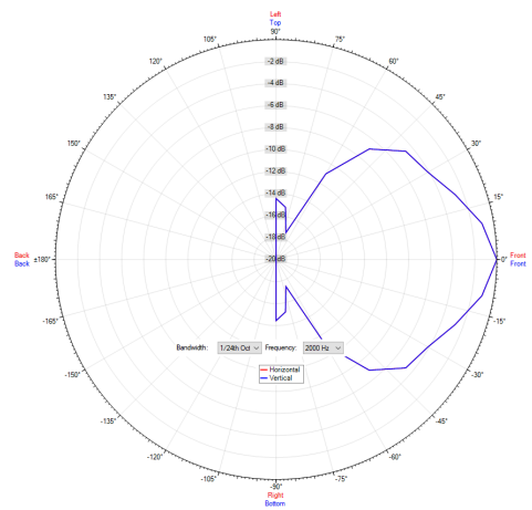
Polardiagramm 2000Hz
