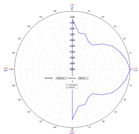
Polardiagramm 1000Hz
