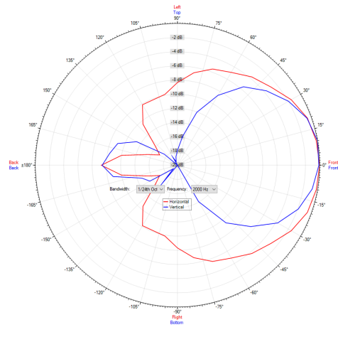
Polardiagramm 2000Hz
