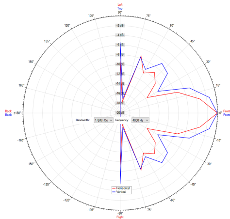
Polardiagramm 4000Hz
