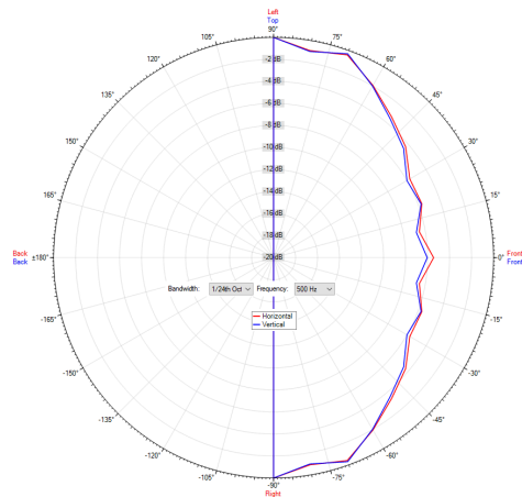
Polardiagramm 500Hz
