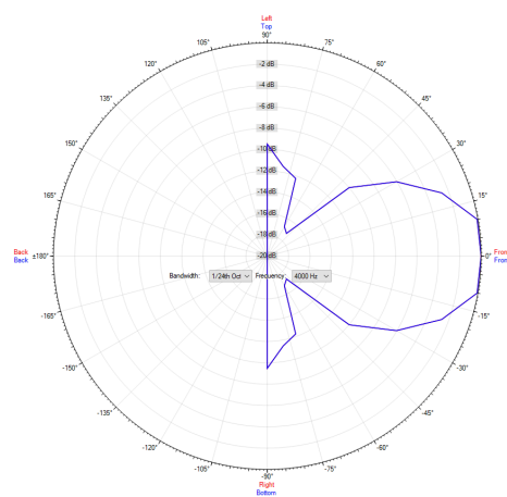
Polardiagramm 4000Hz
