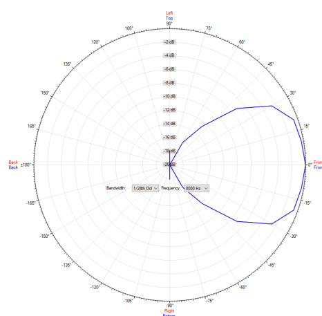
Polardiagramm 8000Hz
