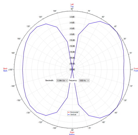
Polardiagramm 1000Hz
