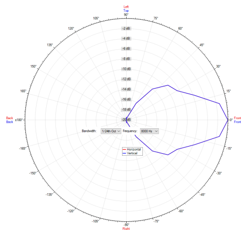
Polardiagramm 8000Hz
