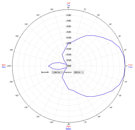
Polardiagramm 2000Hz
