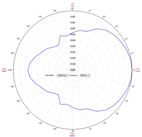
Polardiagramm 1000Hz
