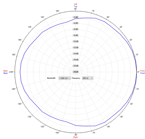
Polardiagramm 500Hz
