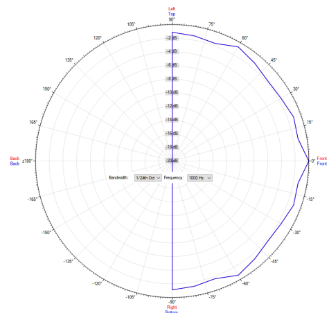
Polardiagramm 1000Hz
