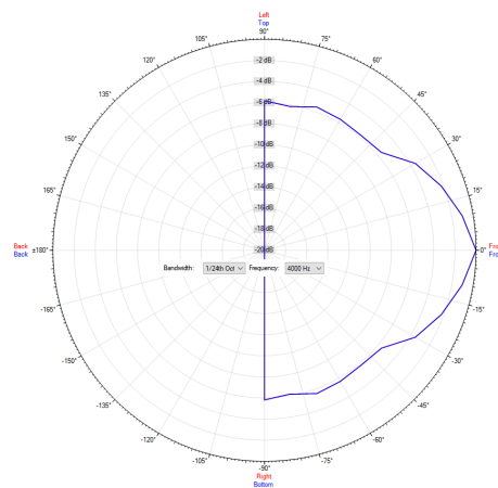
Polardiagramm 4000Hz
