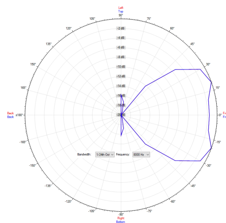
Polardiagramm 8000Hz
