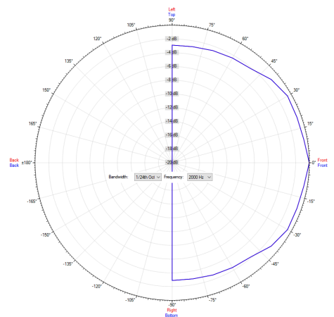
Polardiagramm 2000Hz
