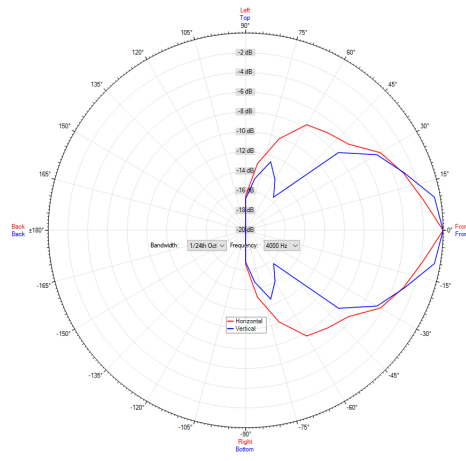
Polardiagramm 4000Hz
