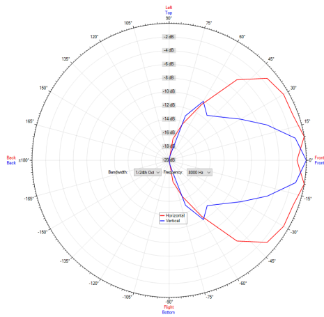
Polardiagramm 8000Hz
