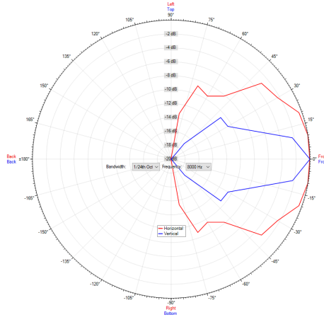
Polardiagramm 8000Hz
