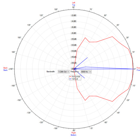
Polardiagramm 8000Hz
