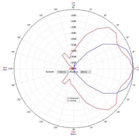
Polardiagramm 4000Hz
