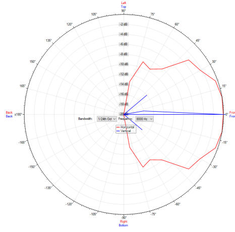
Polardiagramm 8000Hz
