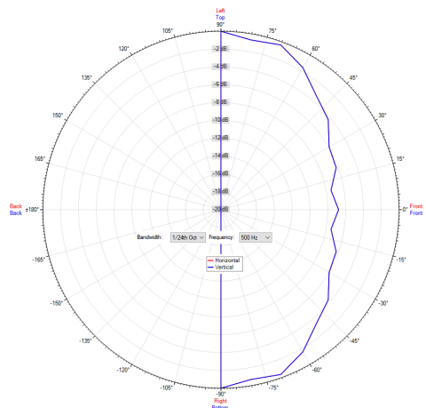
Polardiagramm 500Hz
