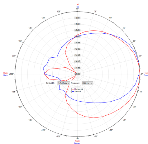
Polardiagramm 2000Hz
